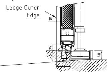
c) Threshold U50D
