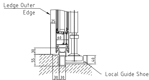
a) Threshold DA
